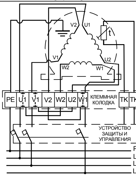
Колеровка проводов питания трёхфазных электродвигателей (-4D; -6D и -8D)
