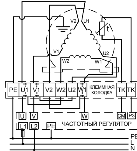
Схема подключения трехфазного электродвигателя вентилятора 90-50/45.4D
