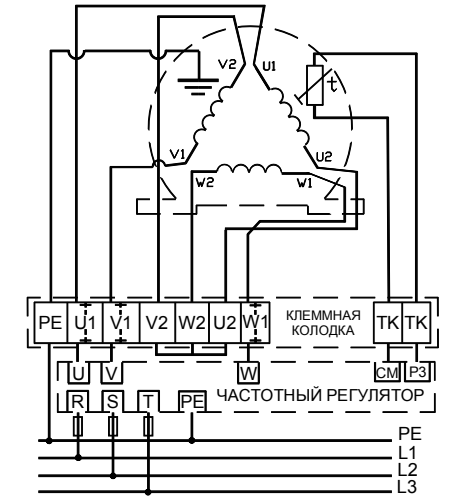
Схема подключения трехфазного электродвигателя вентилятора 90-50/45.4D
